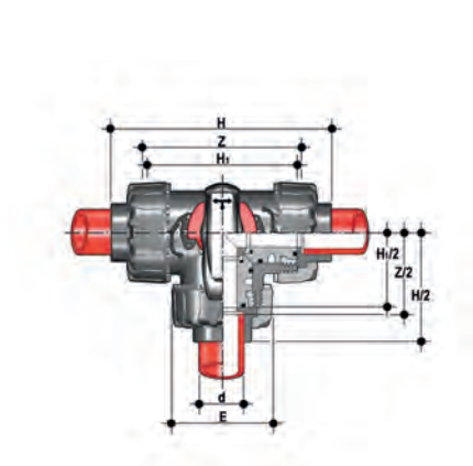
TKDIM Valvola a tre vie DUAL BLOCK® con attacchi femmina per saldatura di tasca, serie metrica sfera a T
