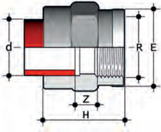
MIMM Manicotto con estremità per saldatura di tasca (d) e con estremità femmina filettata BSP (R) con anello di rinforzo in Acciaio INOX
