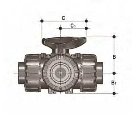
Dimensioni comuni a tutte le versioni
